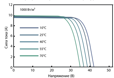
Вольт-амперные характеристики панели при разных рабочих температурах
