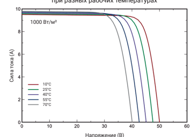
Вольт-амперные характеристики панели при разных рабочих температурах
